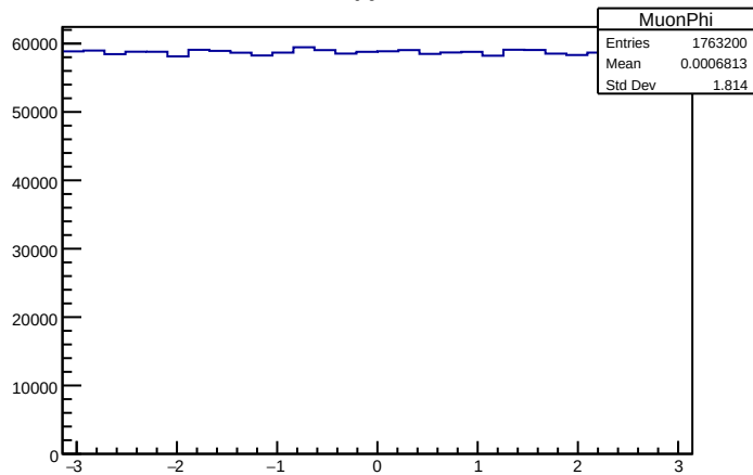
MuonPhi
