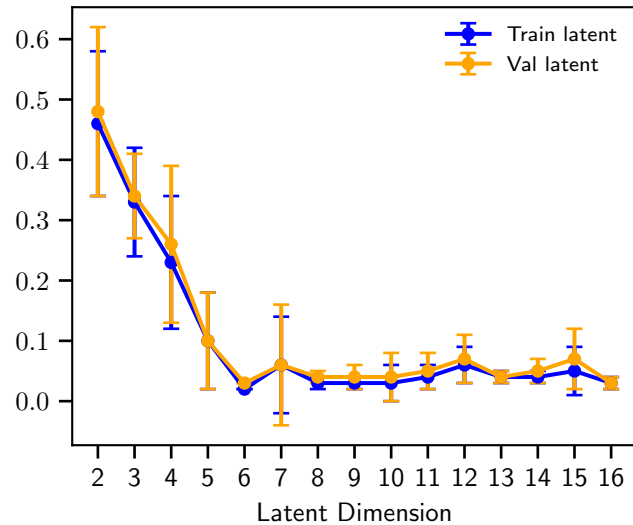
Latent Recon. MAE
