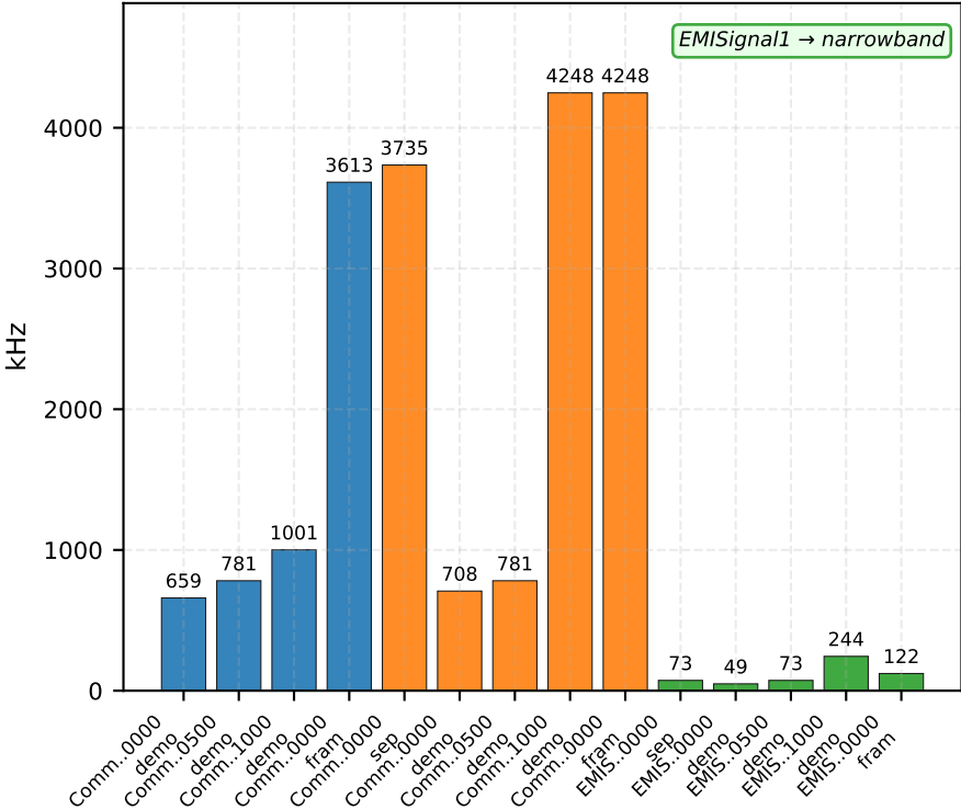
-3 dB Bandwidth (kHz)
