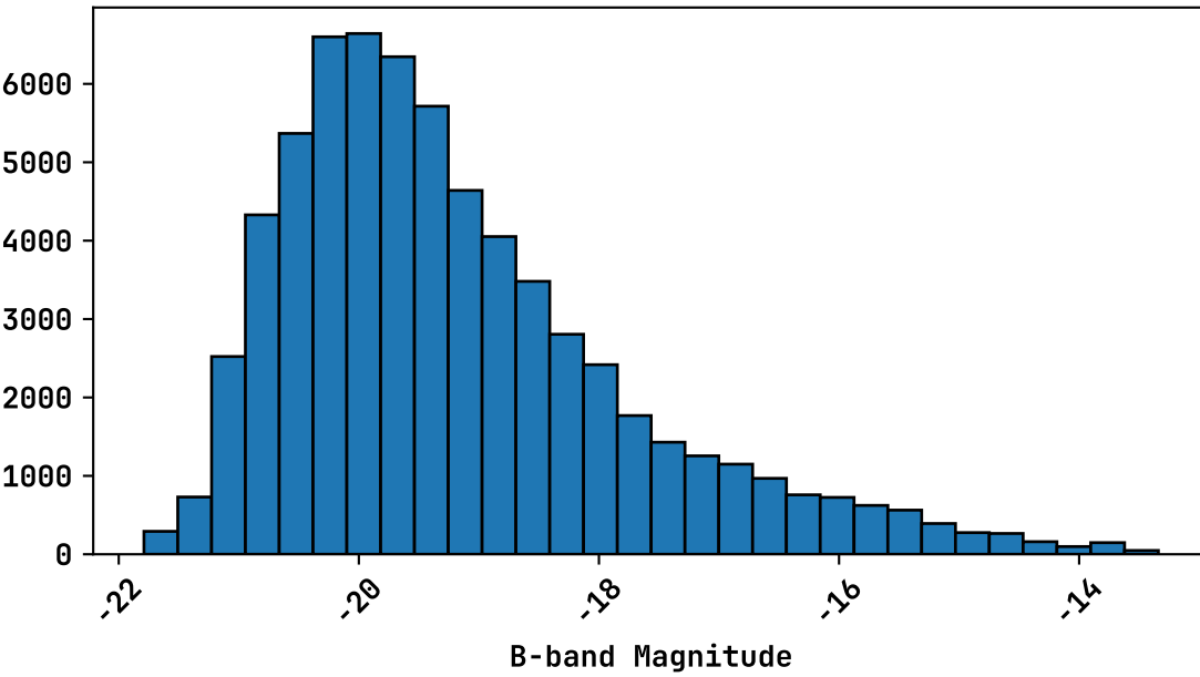
'Filled' GWGC - B-band Magnitude
