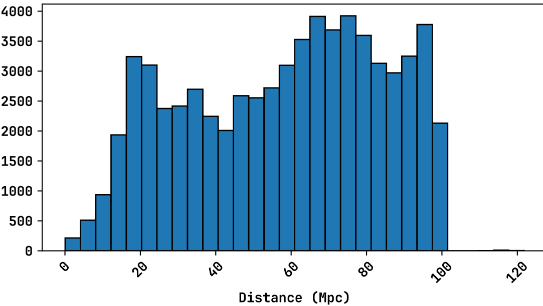
'Filled' GWGC - Distance (Mpc)
