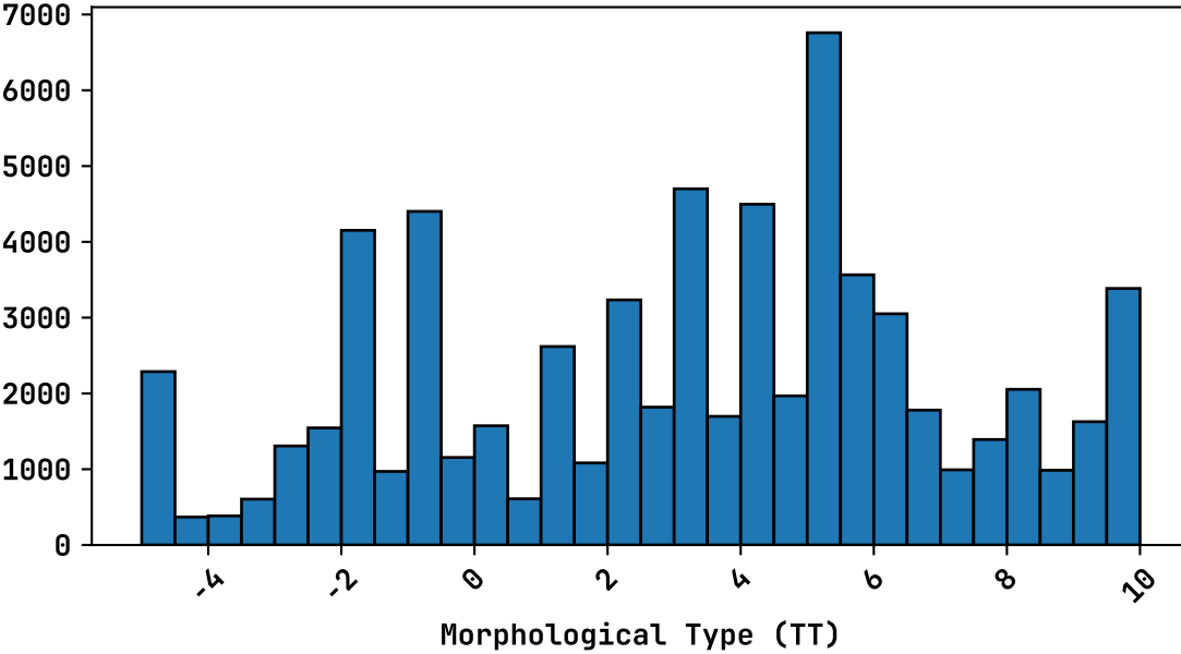
'Filled' GWGC - Morphological Type (TT)
