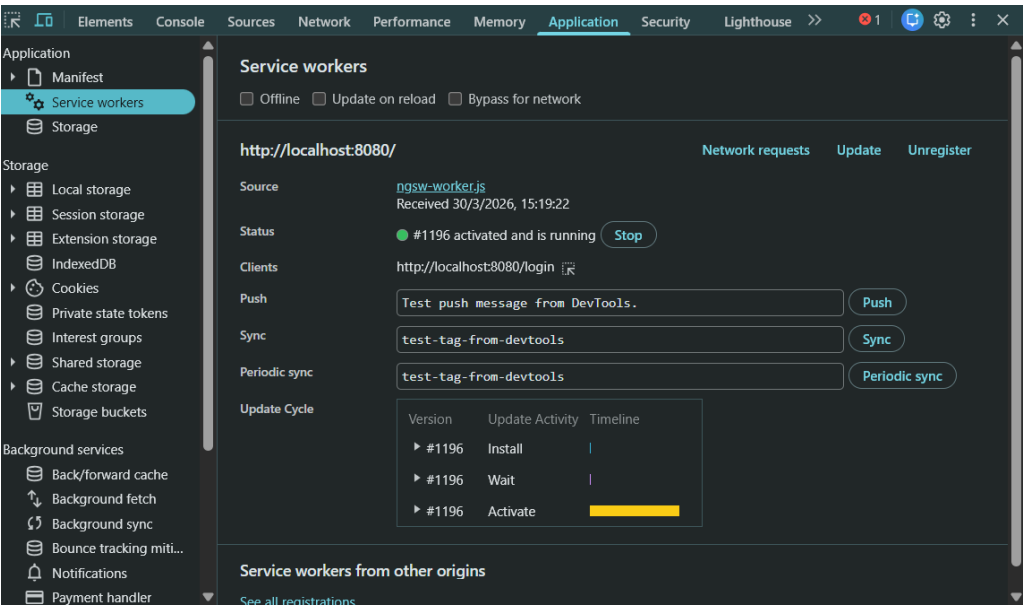
Figura 3: Service worker registrado en herramientas de desarrollo
