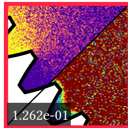
WoSt (4.19s)
