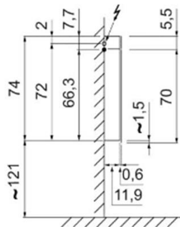
Spiegelschrank
