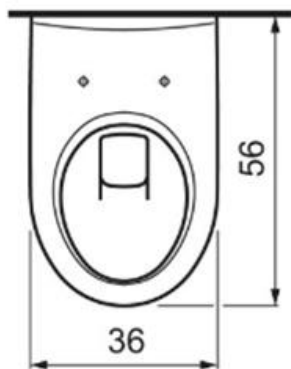
WC Anlage
