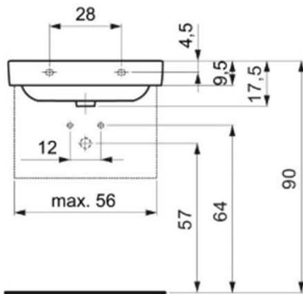
Waschtisch
