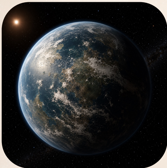
PLANET 5 TOI-700 D
