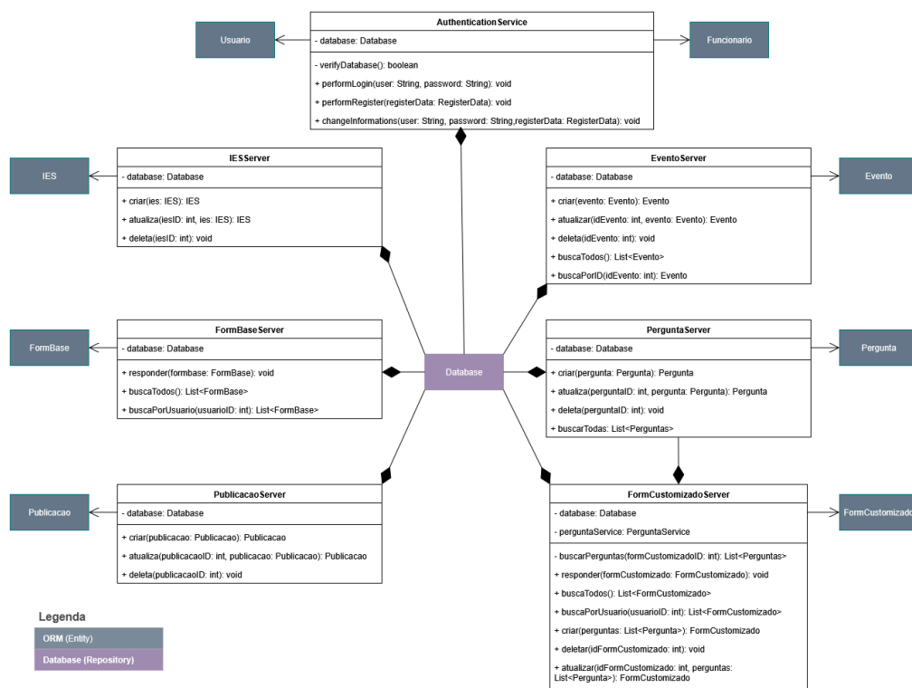
Figura 13 – Diagrama de Classe do projeto.
