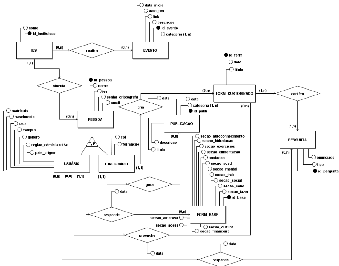
Figura 16 – Diagrama Entidade-Relacionamento do Projeto.
