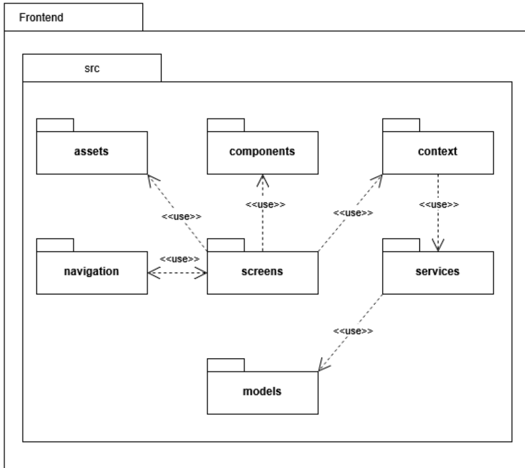
Figura 14 – Diagrama de Pacotes do frontend.
