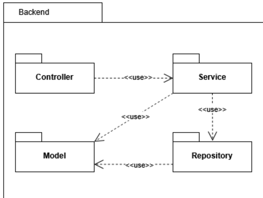
Figura 20 – Diagrama de Pacotes do backend.
