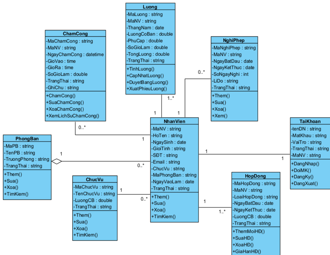
Hình 3.13. Biểu đồ lớp thực thể
