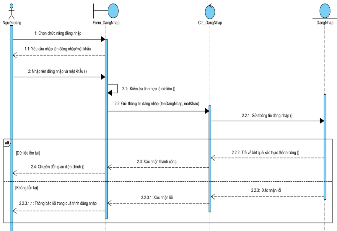
Hình 3.14. Biểu đồ tuần tự chức năng đăng nhập
