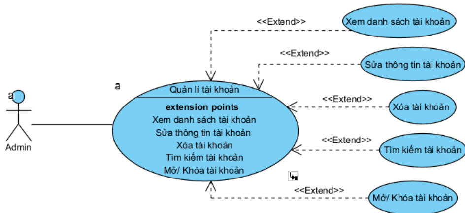
Hình 3.2. Biểu đồ use case Quản lý tài khoản
