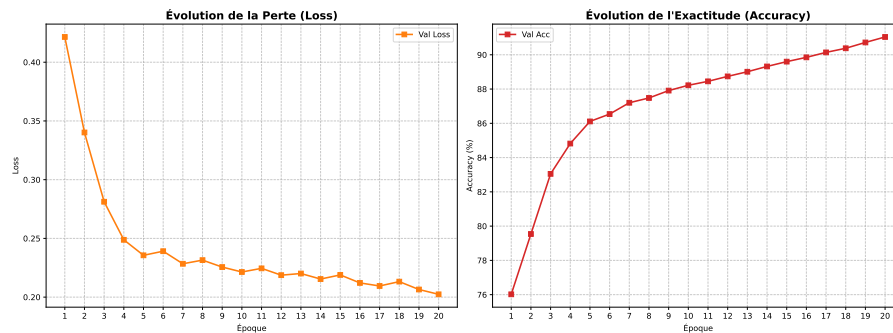
FIGURE 3.1 – Courbes d'apprentissage du modèle
