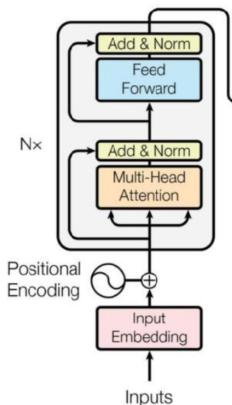
FIGURE 2.4 – Illustration d'un encodeur du papier « Attention is All you Need » (2017)
