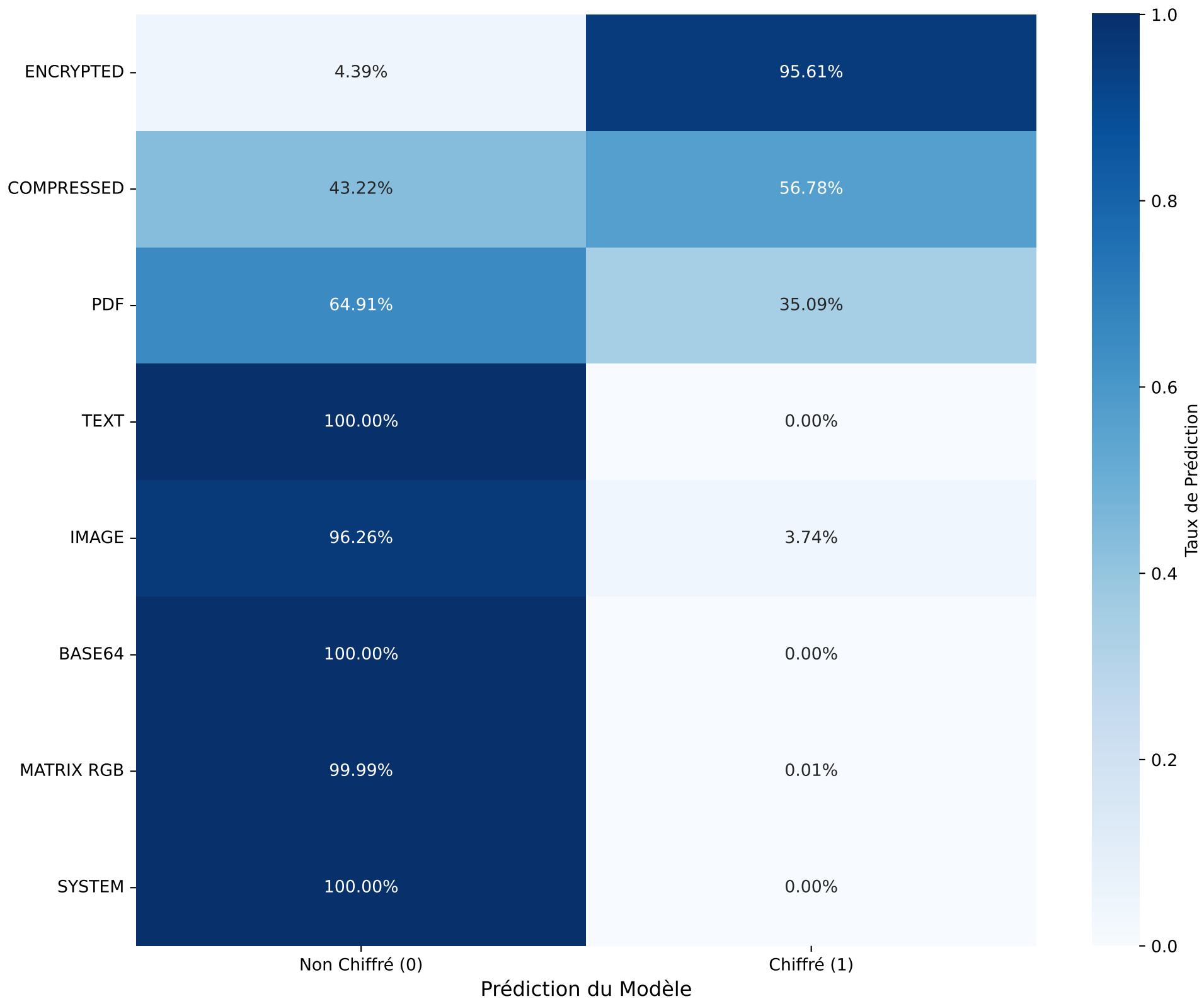
Matrice de Confusion par Sous-Classes
