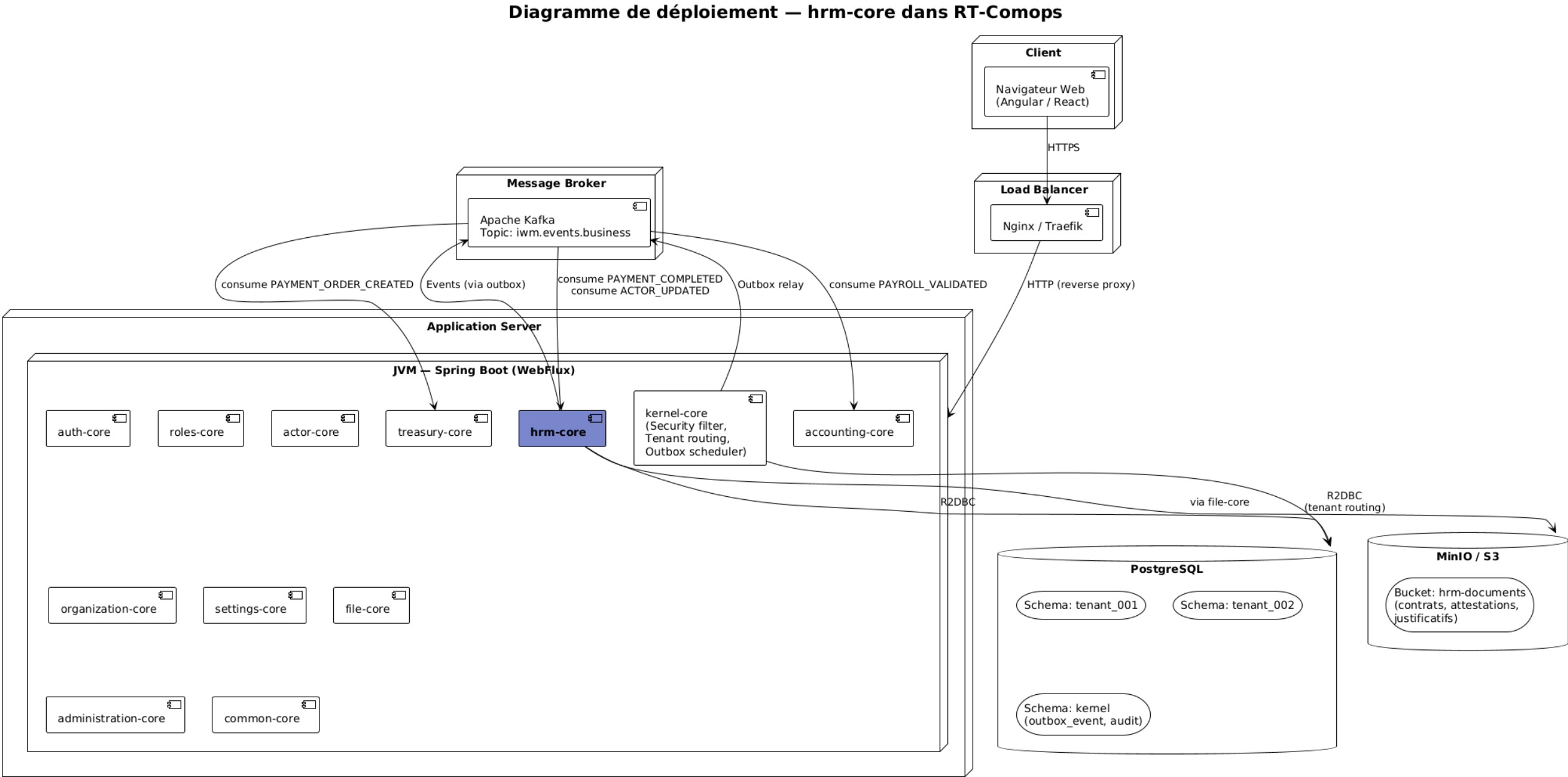
FIGURE 2.5 – Diagramme de déploiement de hrm-core dans l’infrastructure RT-Comops
