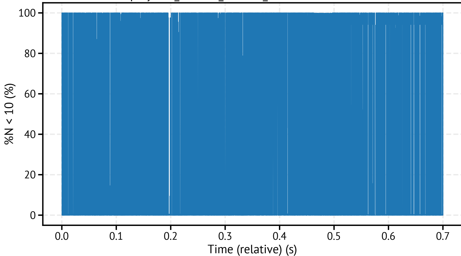
spraytec2_260318_113446_680200.csv - %N < 10
