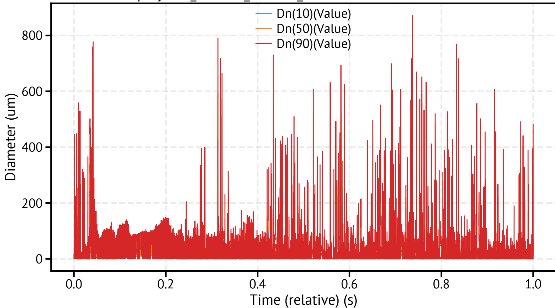
spraytec2_260311_151305_865100.csv - Dn Percentiles
