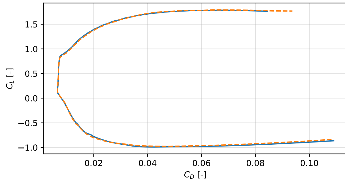
Drag polar
