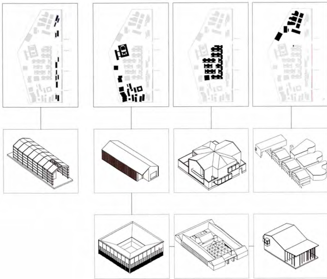
图15 / Figure 15 建筑单体的类型提炼与表达
