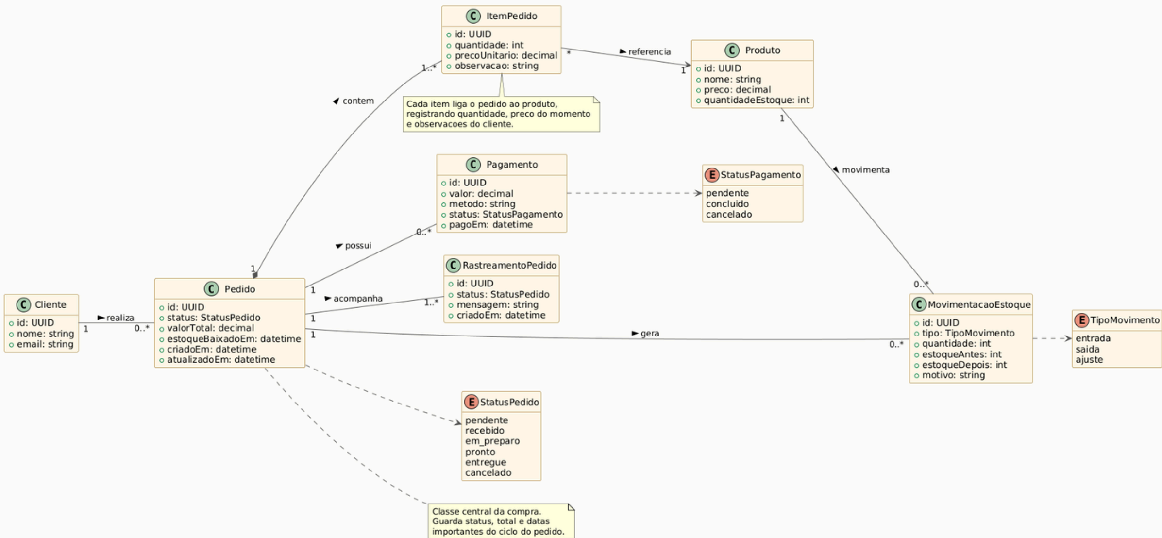
L&J Doces - Diagrama de Classes do Pedido
