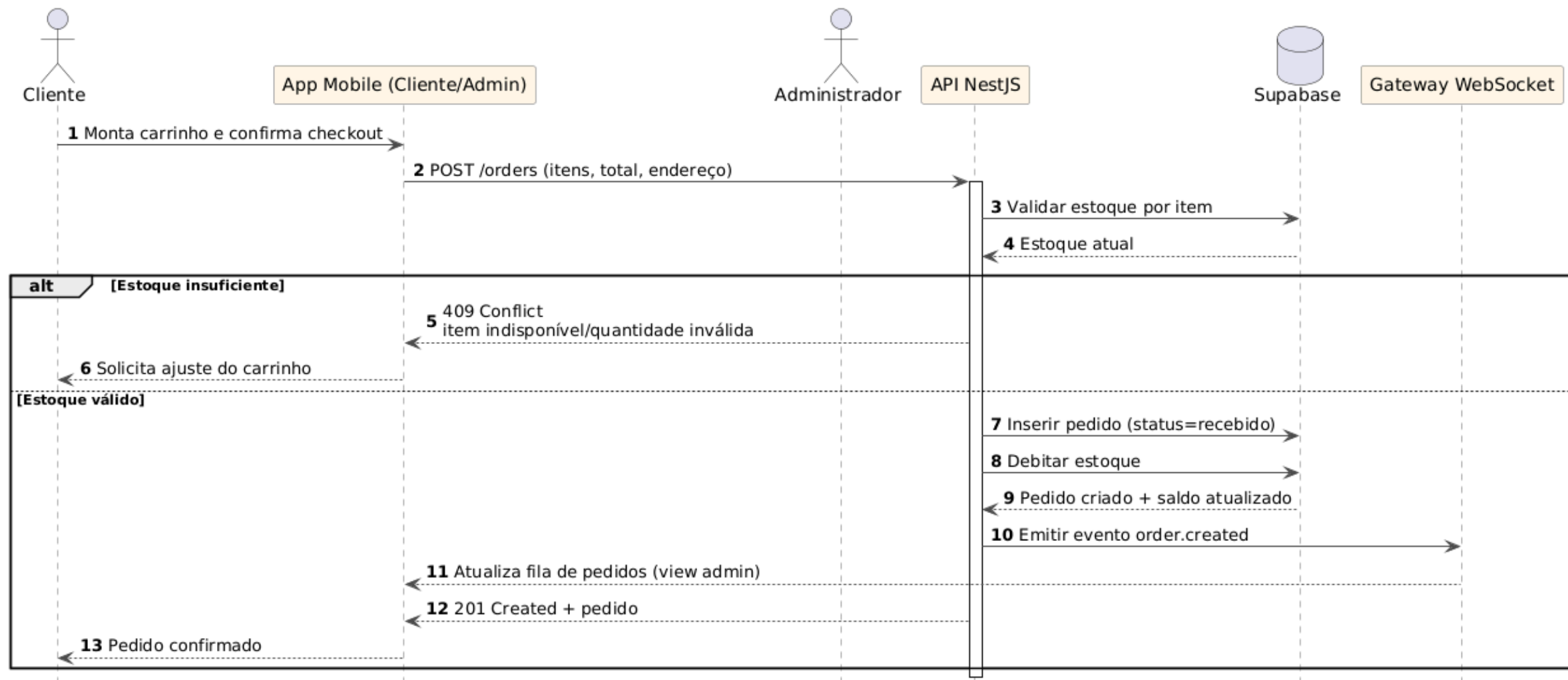
L&J Doces - Fluxo de Pedido (Sequência Detalhada)
