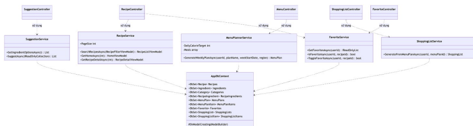
Hình 3.5. Sơ đồ lớp tầng dịch vụ và quan hệ với tầng điều khiển
