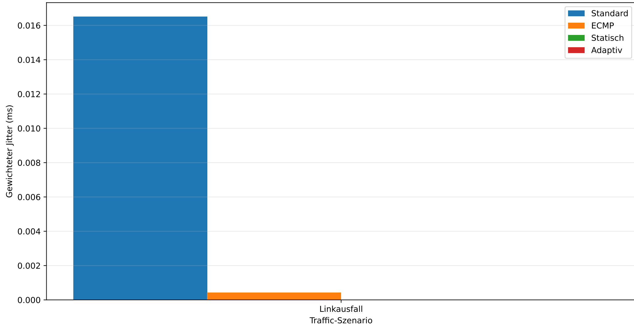
Jitter - Ausfallszenario
