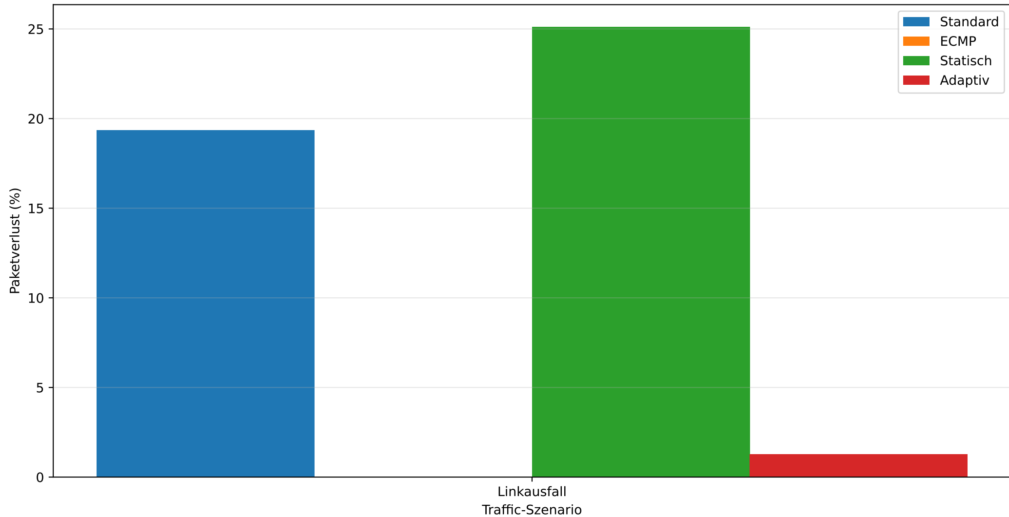
Paketverlust - Ausfallszenario
