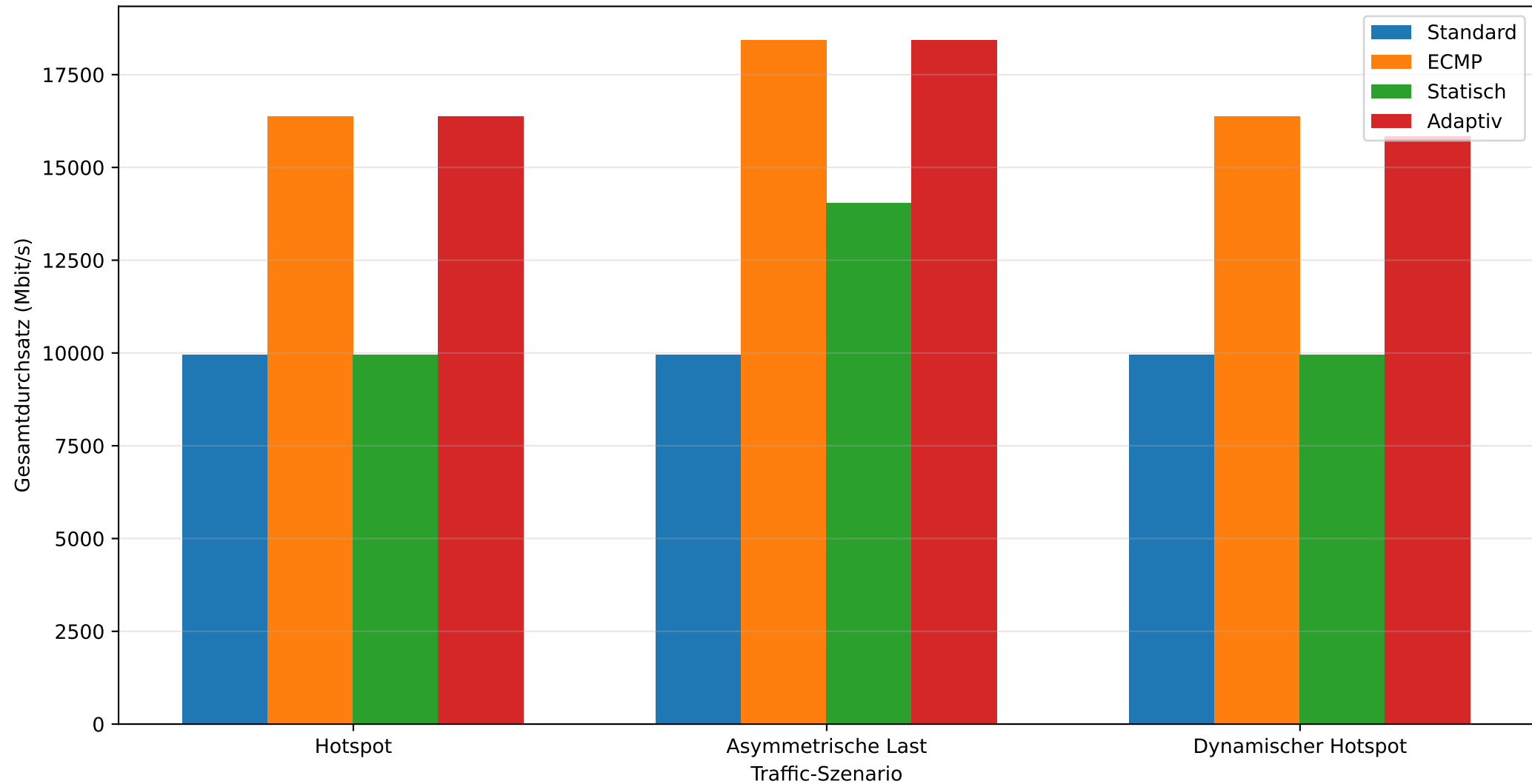
Gesamtdurchsatz - Traffic-Engineering-Szenarien
