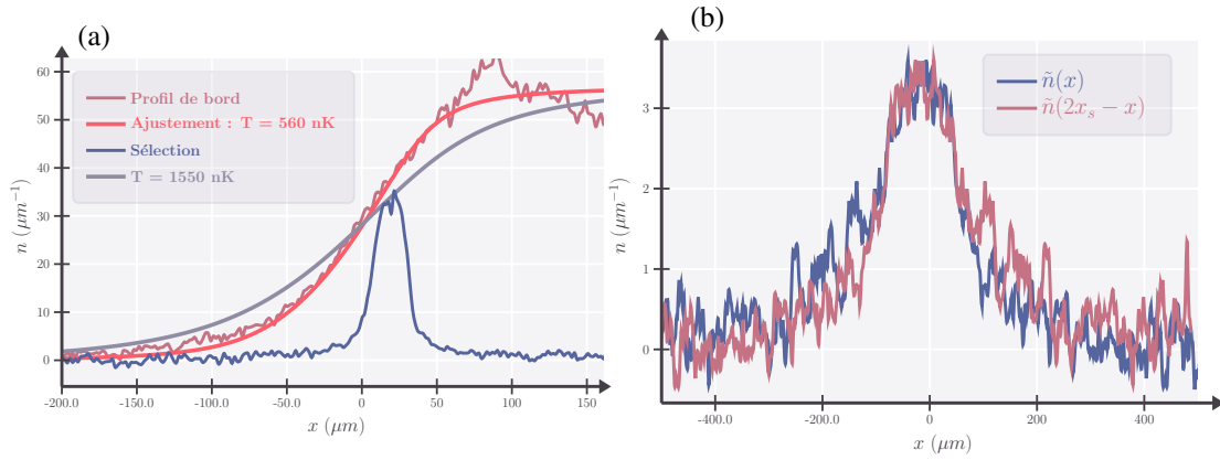
FIGURE 6.2 – (a) Profil de bord et tranche sélectionnée. Le profil de bord après 18 ms est montré en rouge. L'ajustement thermique donne une température T = 560 nK (orange). Le profil de densité mesuré 1 ms après la sélection de la tranche est en bleu. (b) Asymétrie du profil d'expansion de la tranche. Le profil de densité après une expansion pendant \tau = 30 ms est comparé à son image miroir. Le centre de symétrie x_s = -17 \mu\text{m} minimise la distance quadratique \delta^2(x_s) = \int dx \left[ \frac{\tilde{n}(x) - \tilde{n}(2x_s - x)}{2} \right]^2 / \int dx n(x)^2 .
