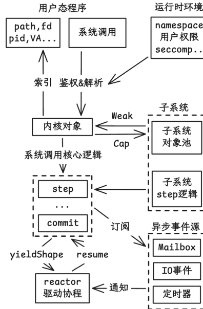
图 8 txKernel 的核心设计。左侧是系统调用的主轴，以对象解析和协程执行为核心；右侧是内核完成 POSIX/Linux 语义的子系统。整个子系统的设计围绕系统调用的工作流程和核心抽象所展开。
