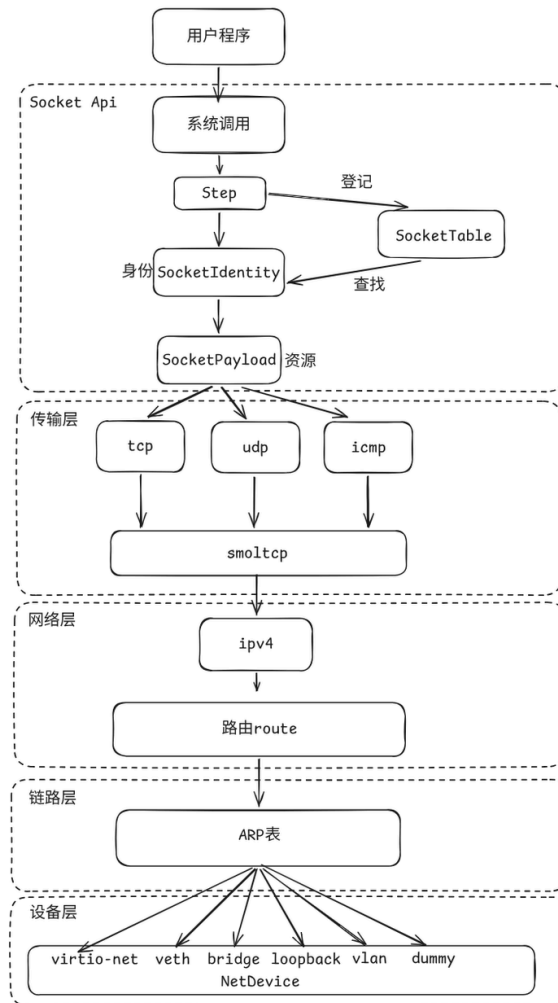
图 24 网络栈概述
