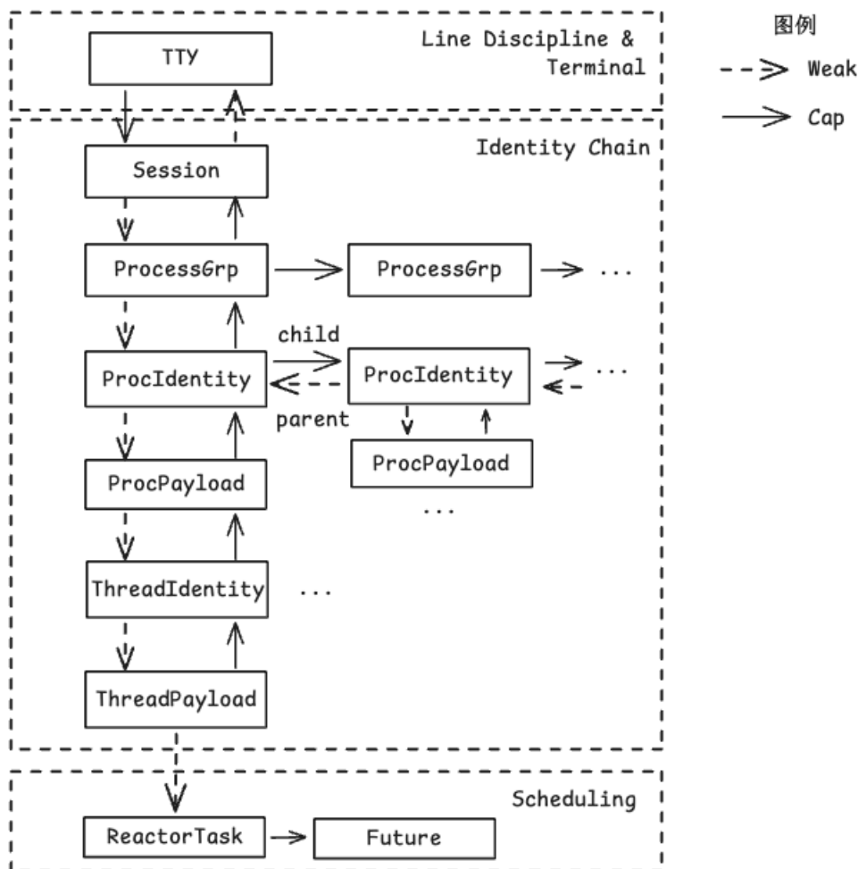
图 14 进程管理整体架构图
