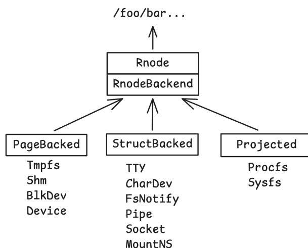
图 7 Rnode 的三大后端和支持的子系统。只有左侧的子系统需要用到 inode 作为页缓存容器的功能。
