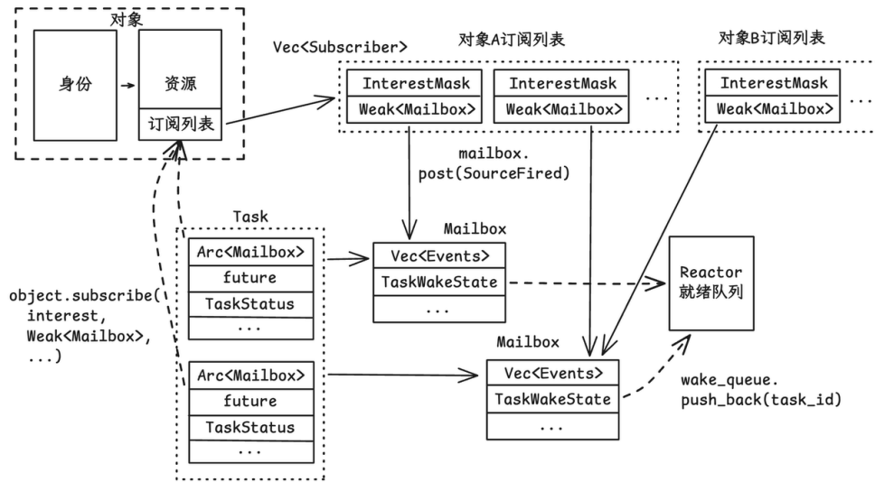
图6 txKernel 的消息传递架构。Vec 实现了 1:N 的通知；Task 可以生成多个 Weak，注册到不同对象的订阅链表里，实现了 1:M 的订阅。
