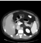
ADMM-TV
