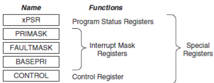
图 3-3Cortex-M 系列的特殊功能寄存器
