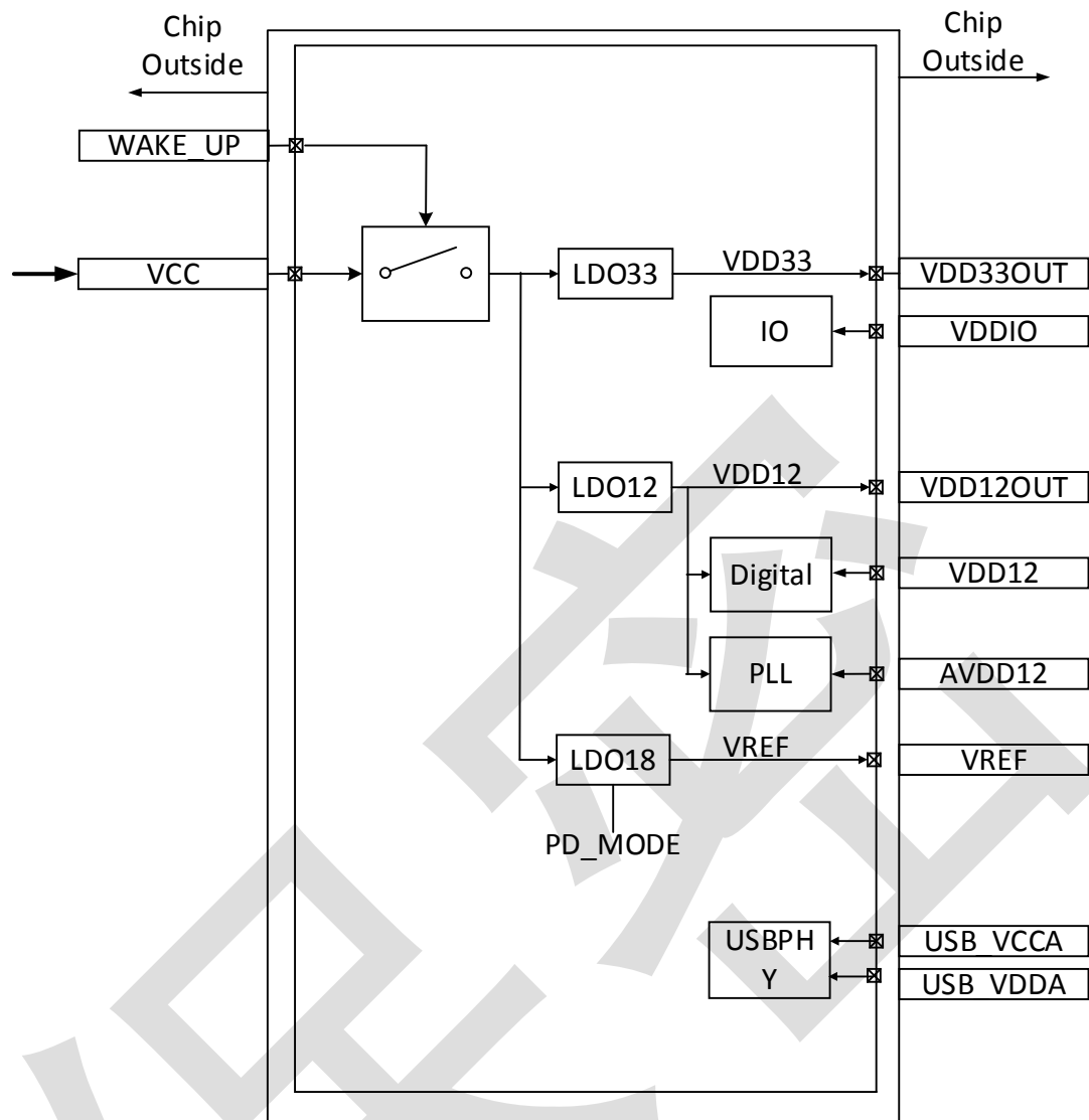
图 1-2 电源框图
