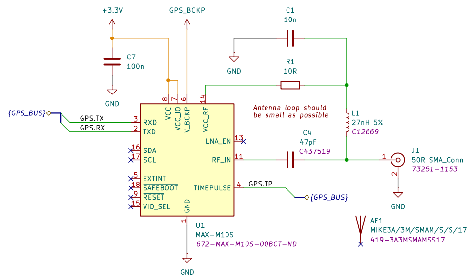
GPS Module
