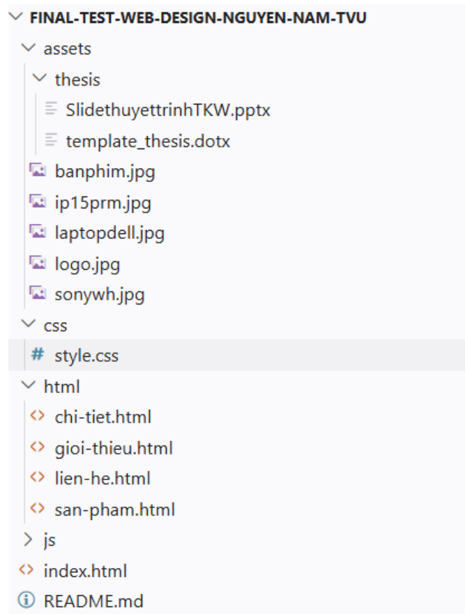
Hình 3.1: Sơ đồ cây thư mục dự án TechStore
