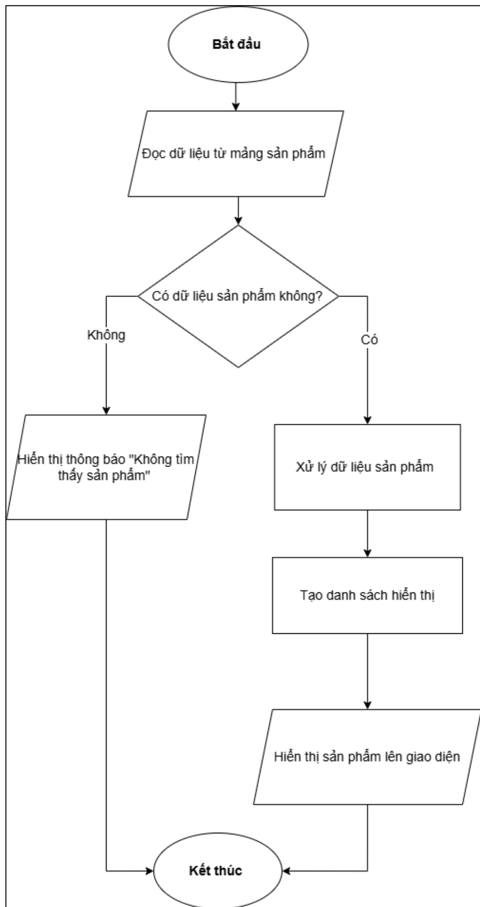
Hình 3.5. Sơ đồ khối chức năng hiển thị sản phẩm
