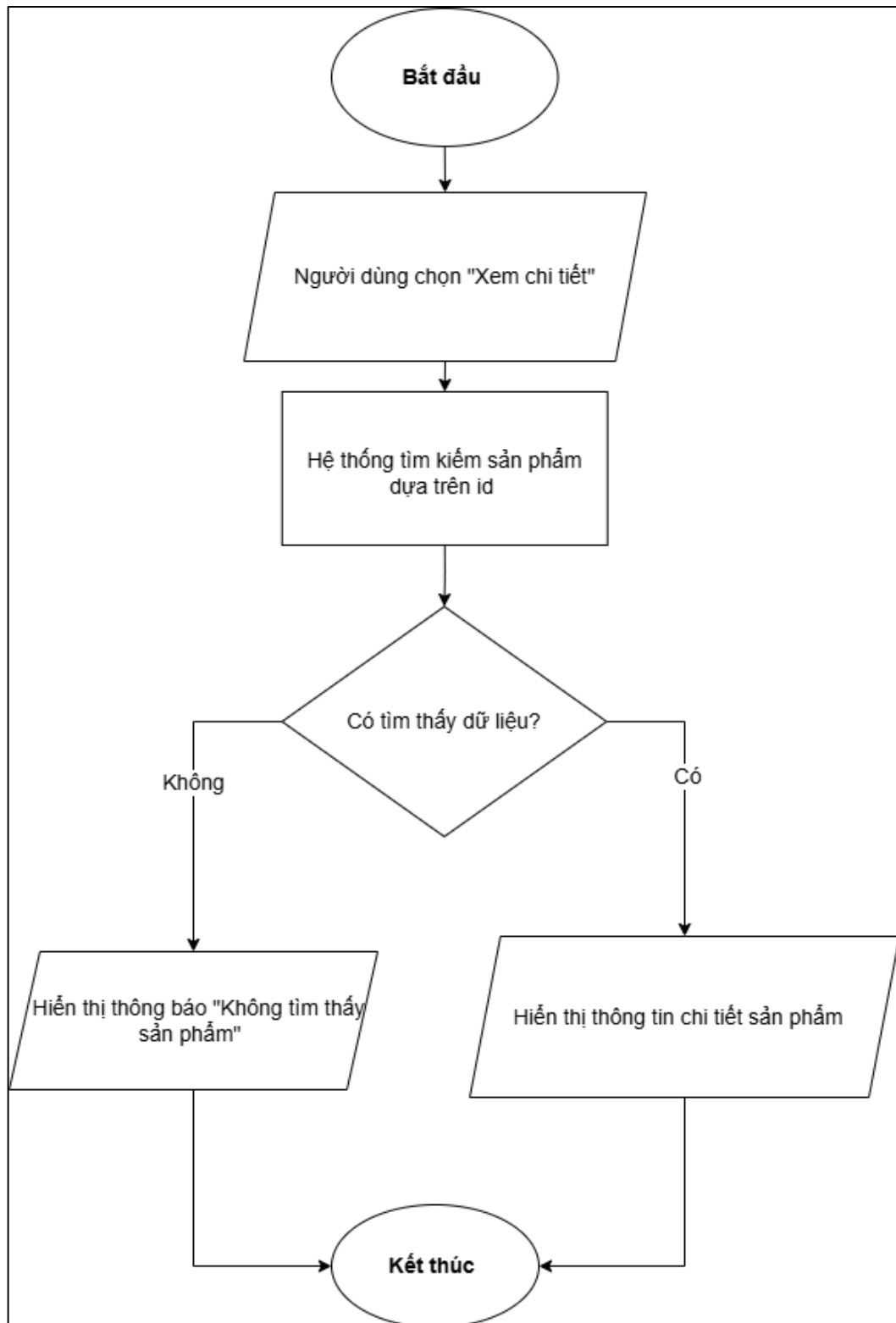
Hình 3.8. Sơ đồ khối chức năng xem chi tiết sản phẩm
