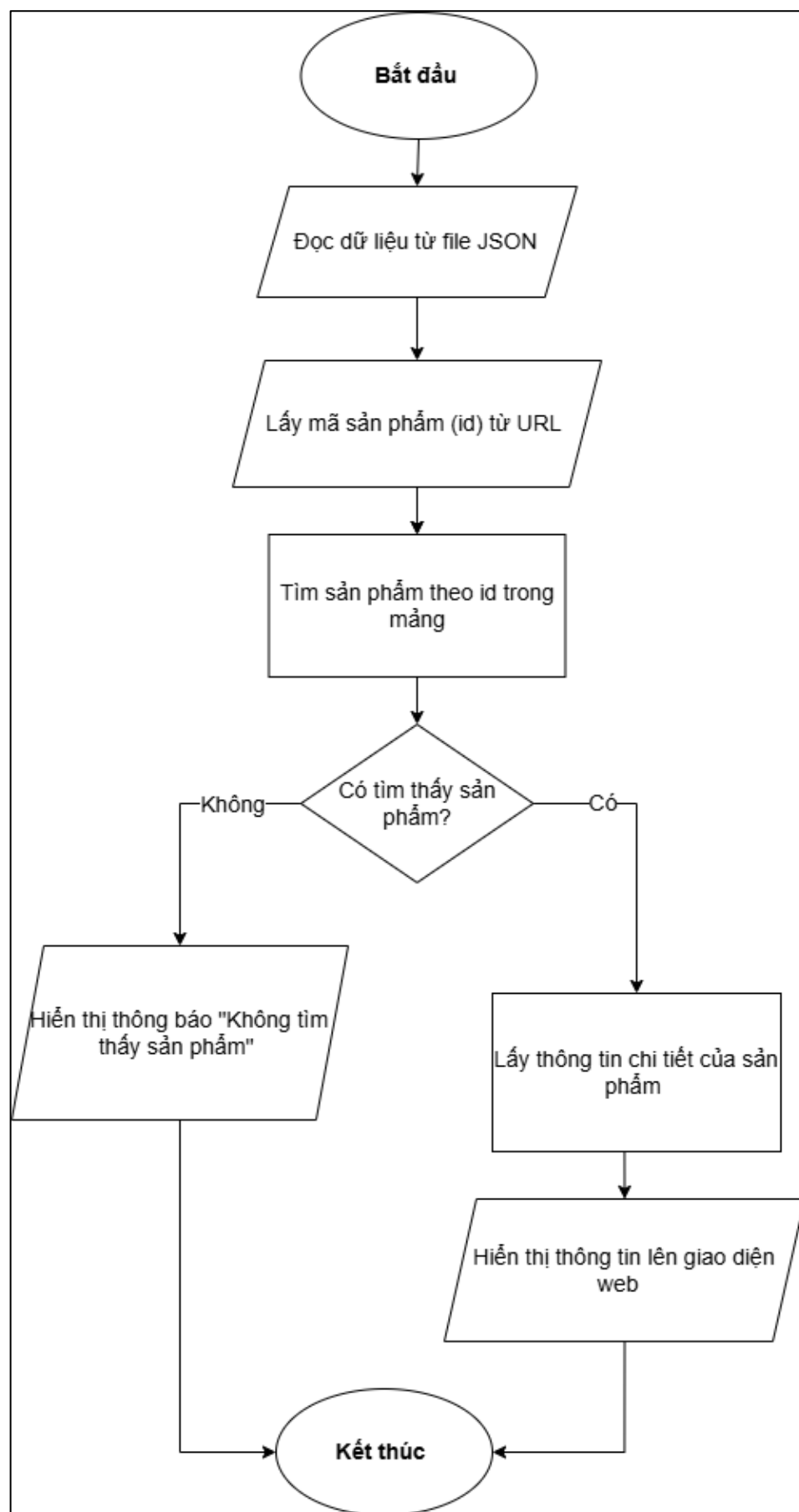
Hình 3.4. Sơ đồ khối đặc tả thuật toán xem chi tiết
