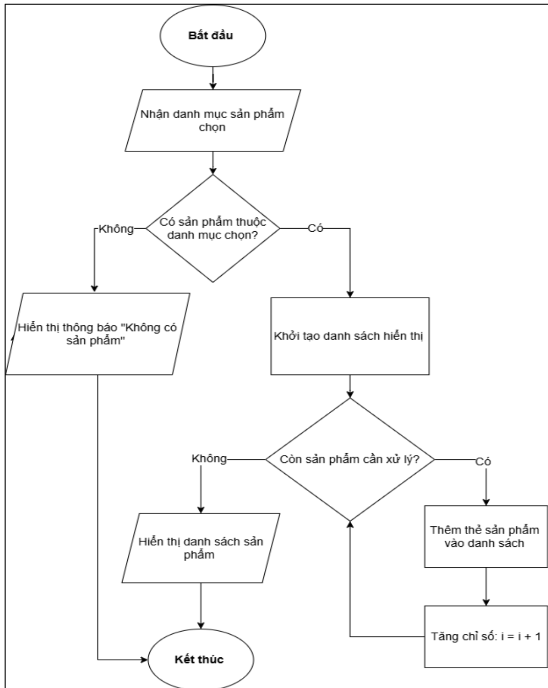
Hình 3.3. Sơ đồ đặc tả thuật toán lọc sản phẩm theo danh sách
