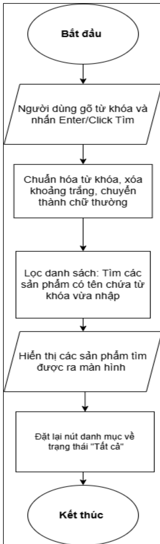
Hình 3.2. Sơ đồ khối đặc tả thuật toán tìm kiếm
