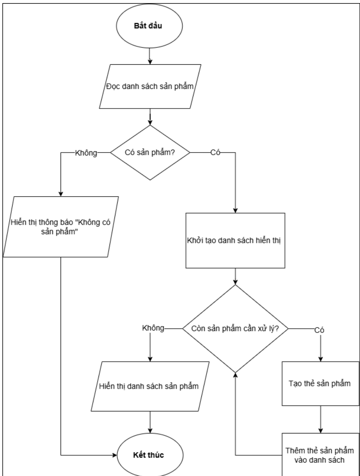
Hình 3.1. Sơ đồ khối đặc tả thuật toán hiển thị
