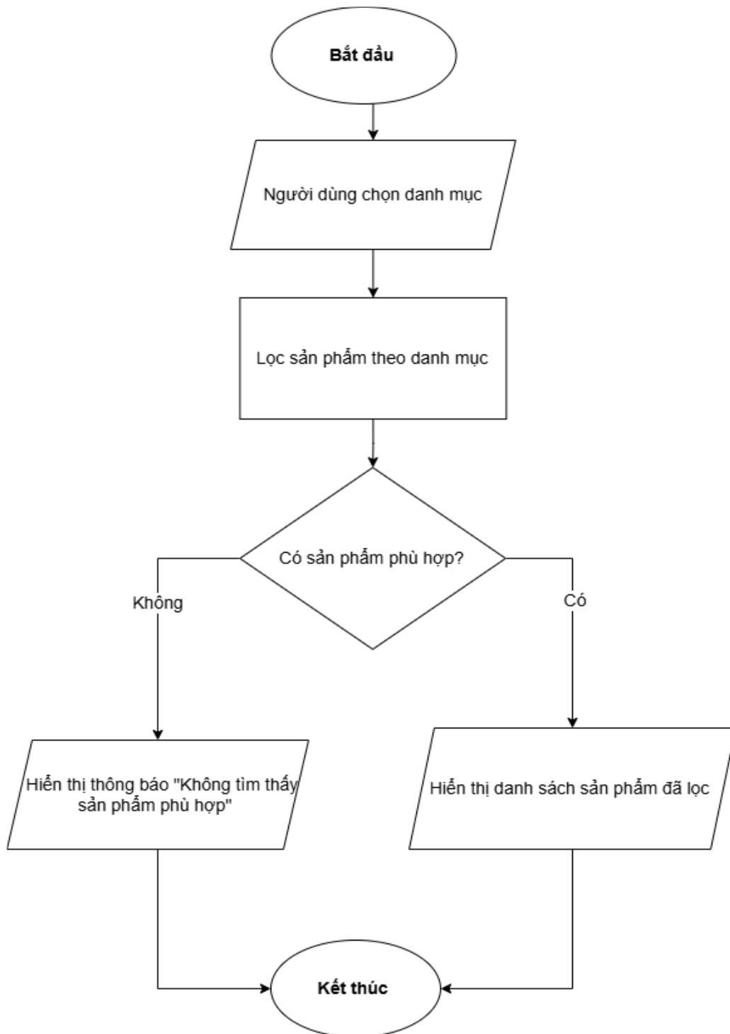
Hình 3.6. Sơ đồ khối chức năng phân loại sản phẩm
