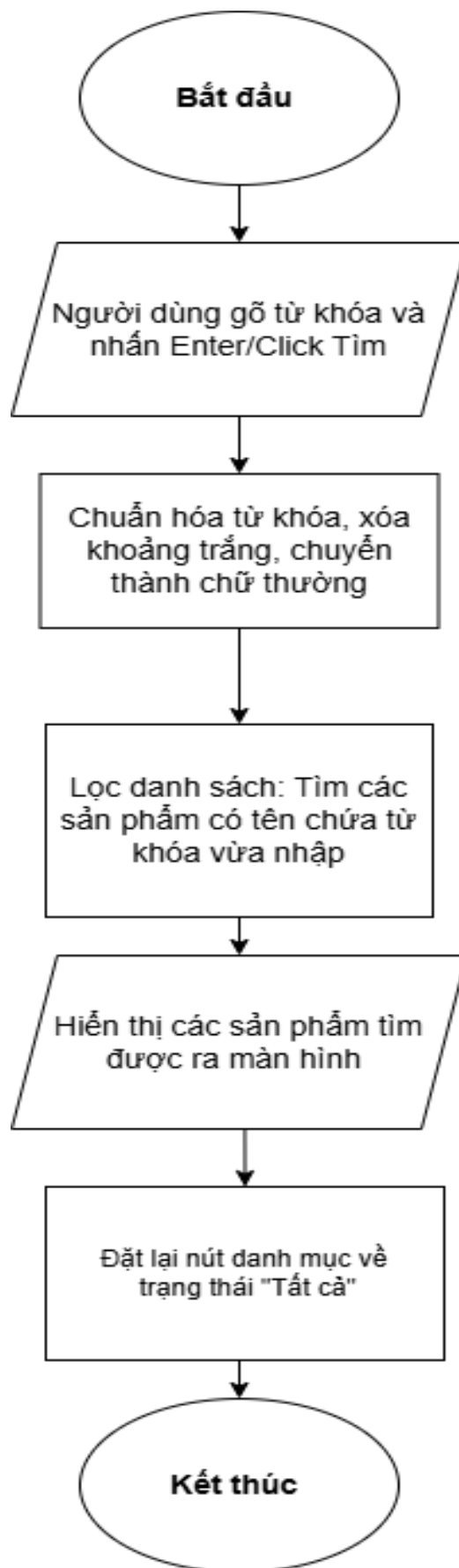
Hình 3.2. Sơ đồ khối đặc tả thuật toán tìm kiếm
