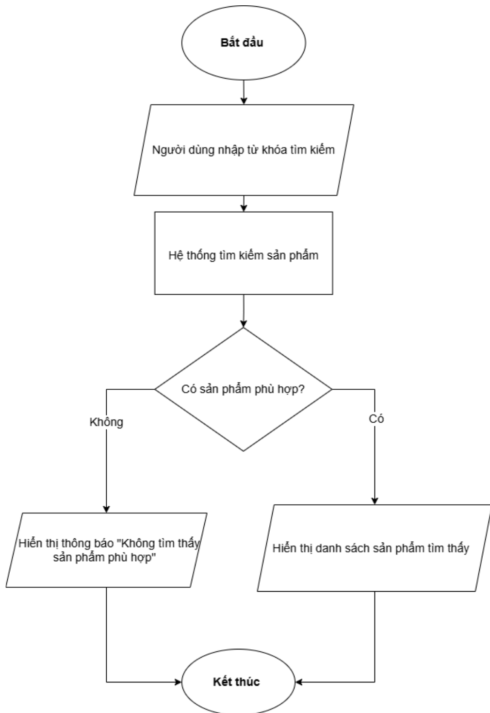
Hình 3.7. Sơ đồ khối chức năng tìm kiếm sản phẩm
