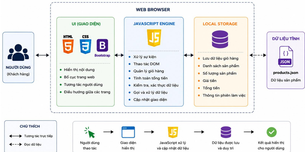
Hình 3.5 Kiến trúc hoạt động của hệ thống
