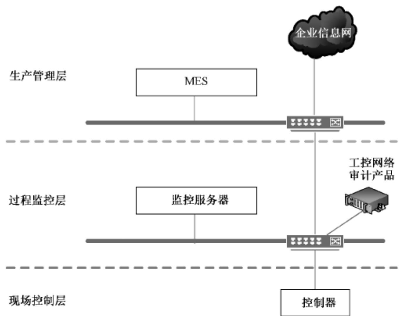
图 A.1 一体式工业控制系统网络审计产品典型部署示意图
