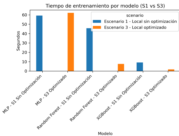
Figura 7. Tiempo de entrenamiento por modelo (Escenario 1 vs Escenario 3)
