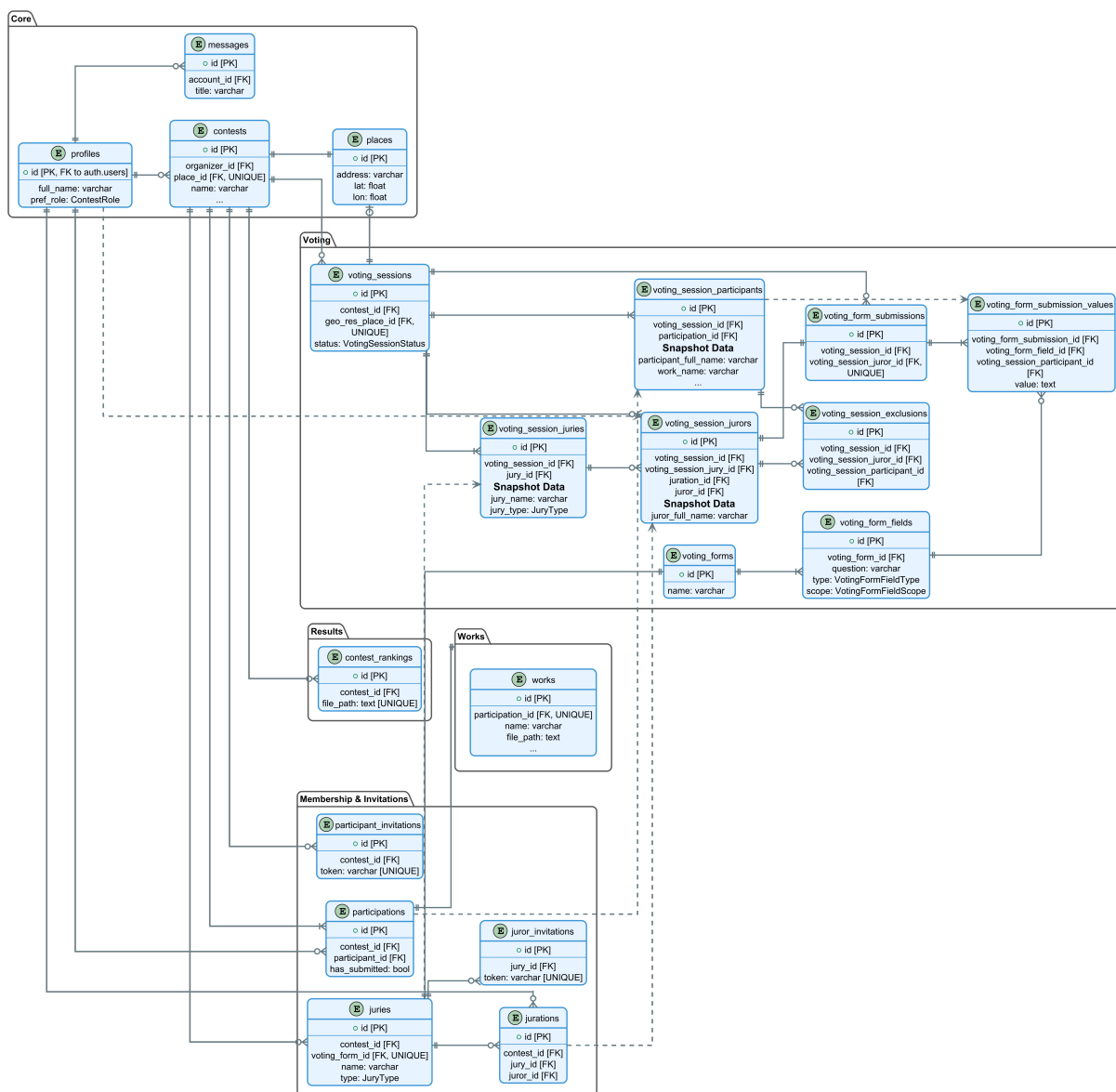
Figura 4.3: Diagramma Entità-Relazioni (ERD) dello schema del database.
