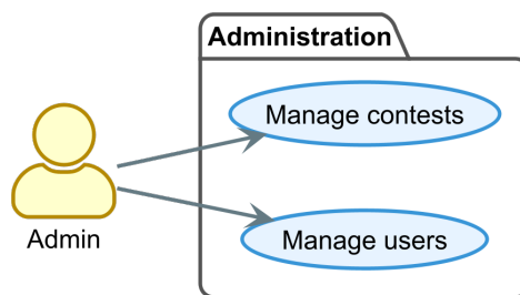
Figura 2.5: Diagramma dei Casi d'Uso: Amministrazione del Sistema.
