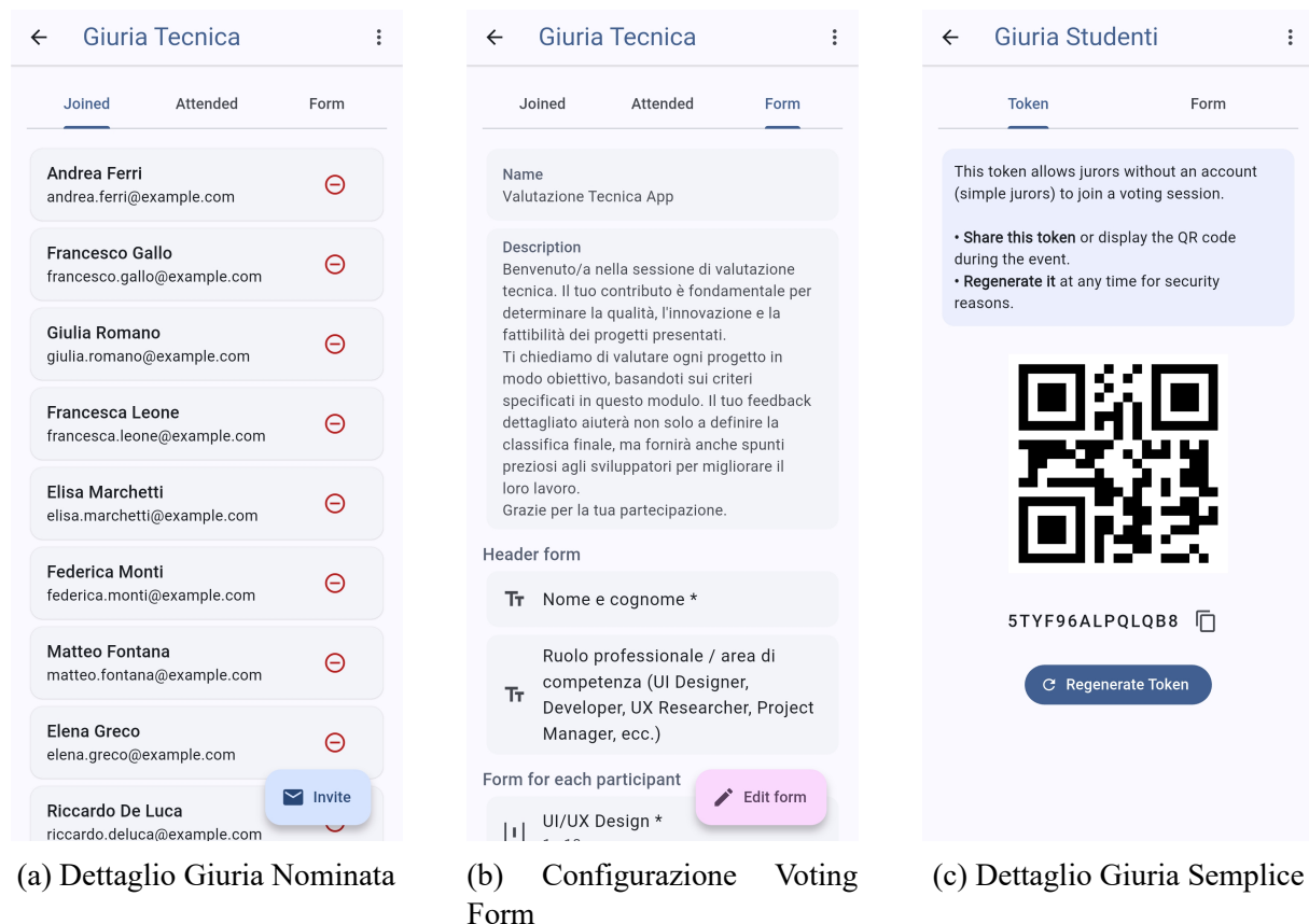
Figura 5.9: Le viste di dettaglio per i due tipi di giuria e la schermata di configurazione del Voting Form associato.
