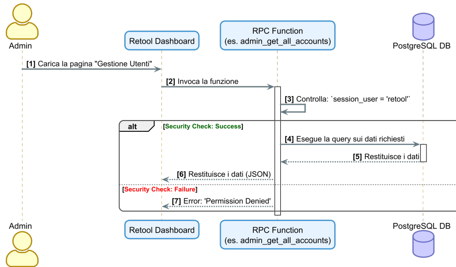
Figura 4.4: Flusso di una chiamata sicura da Retool a una Funzione RPC.
