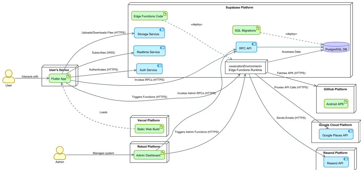
Figura 5.1: Diagramma di distribuzione dell'architettura completa di Swift Contest.
