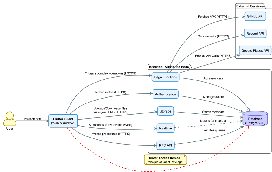
Figura 4.1: Architettura Client-Server del sistema Swift Contest con backend BaaS.
