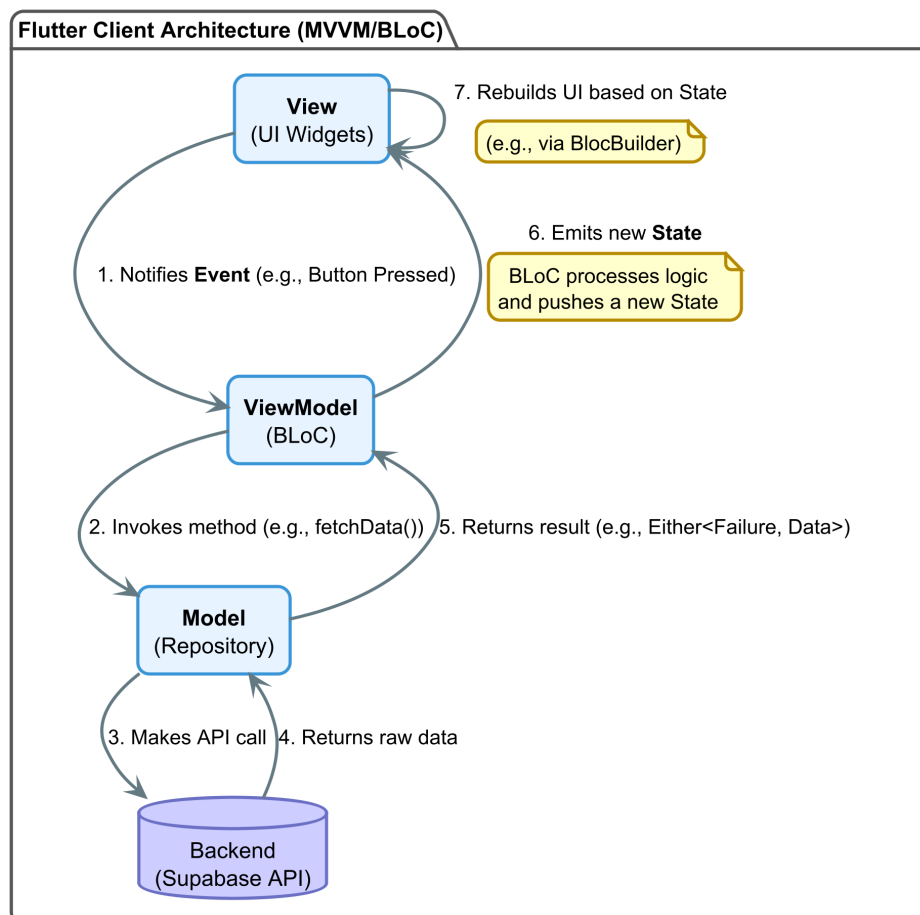
Figura 4.2: Architettura del Client MVVM con BLoC.
