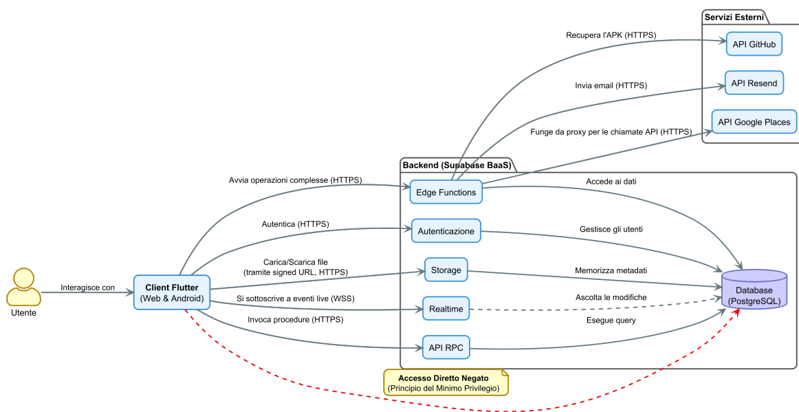
Figura 4.1: Architettura Client-Server del sistema Swift Contest con backend BaaS.
