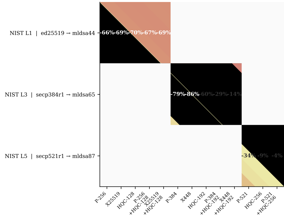
TLS
