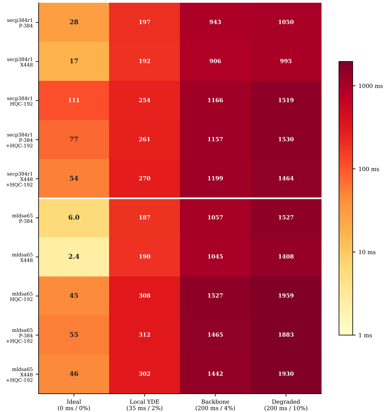
TLS
