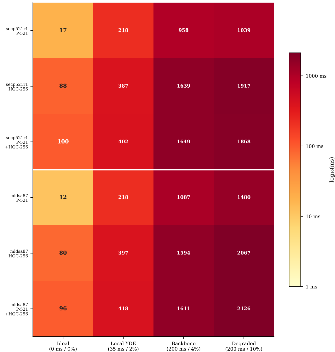
TLS
