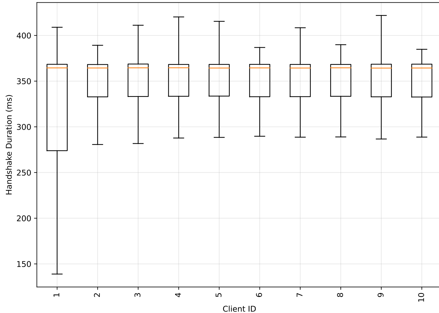
Distribution par client — mldsa65 × hqc192
