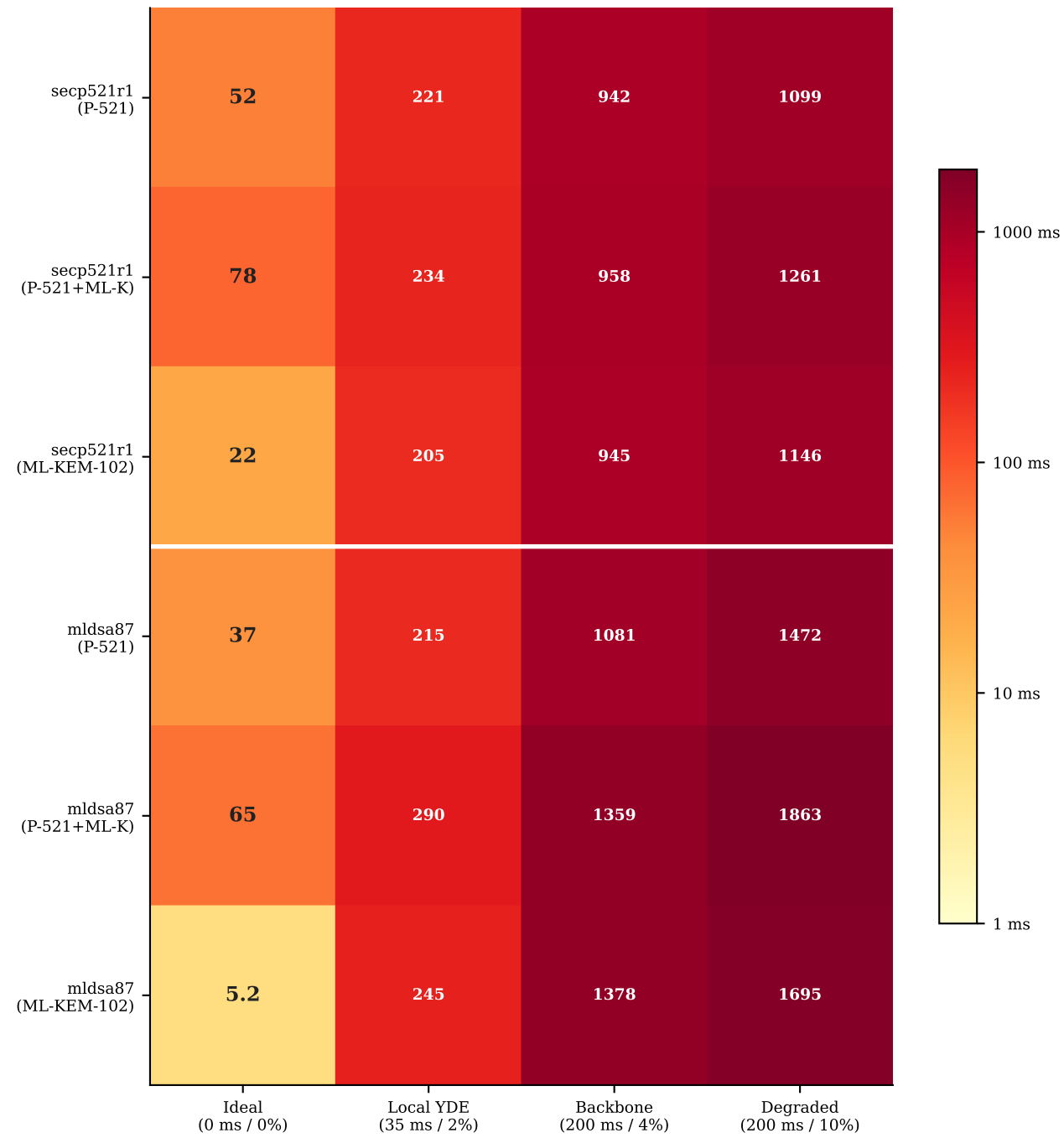
TLS
