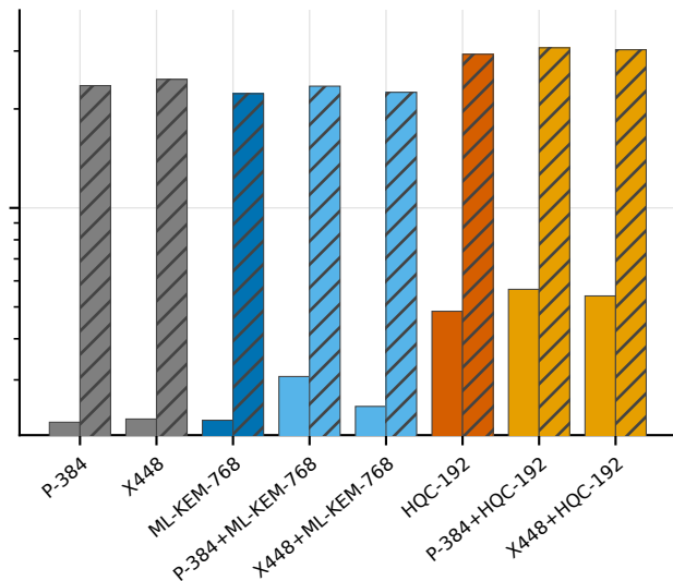
mldsa65 (post-quantum)
