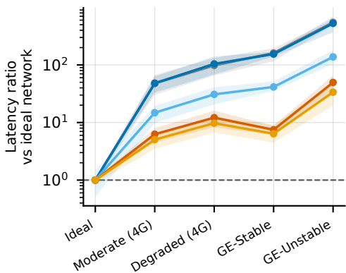
(d) L1 - QUIC
