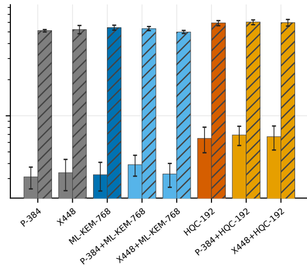
mldsa65 (post-quantum)
