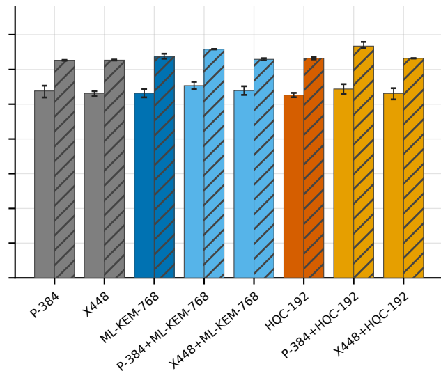
mlDSA65 (post-quantum)
