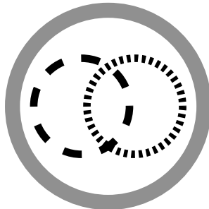
CounterSat CSA
