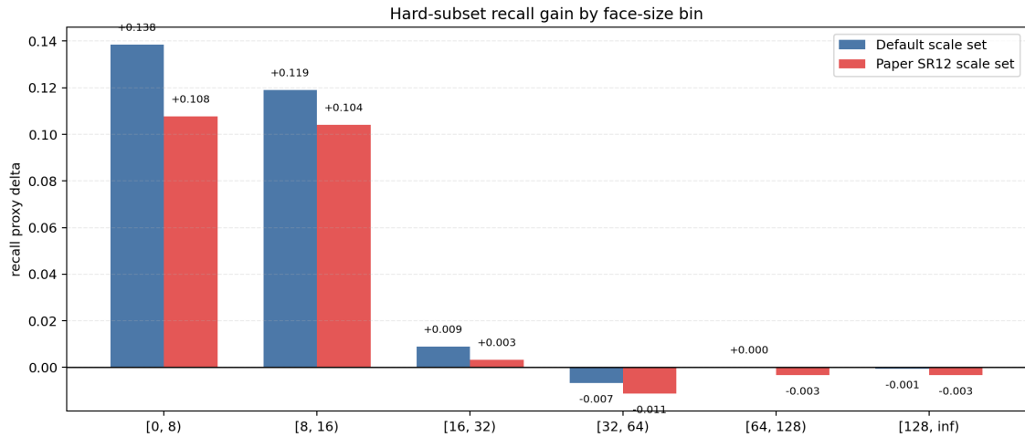
Hình III.6: Mức tăng khả năng thu hồi trên tập Hard theo từng khoảng kích thước khuôn mặt.
