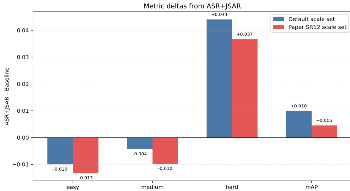
Hình III.4: Mức tăng hoặc giảm của mô hình cải tiến so với mô hình gốc trên từng chỉ số đánh giá.
