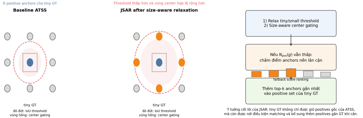
Hình III.2: Nguyên lý của cơ chế phân phối lại phép gán mẫu. Trái: gán nhãn ban đầu thường cho quá ít anchor dương với khuôn mặt rất nhỏ. Giữa: nối điều kiện chấp nhận theo kích thước. Phải: bổ sung một số anchor gần nhất nếu số anchor dương vẫn còn quá ít.
