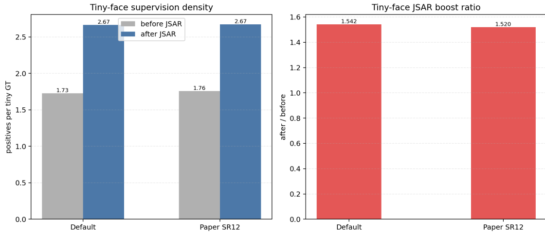
Hình III.5: Mật độ anchor dương trên mỗi khuôn mặt rất nhỏ trước và sau khi áp dụng cơ chế gán nhãn cải tiến.
