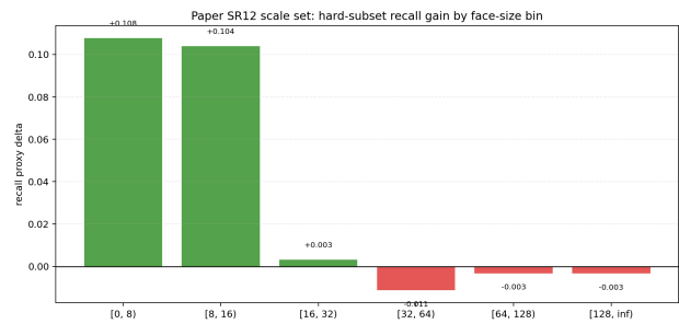
(b) Bộ 12 mức theo bài báo
