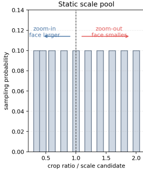
Trước ASR, mỗi crop ratio được lấy gần như đồng đều. Với pipeline SCRFD, scale lớn hơn tương ứng với crop rộng hơn và ảnh mật nhỏ hơn sau resize.
