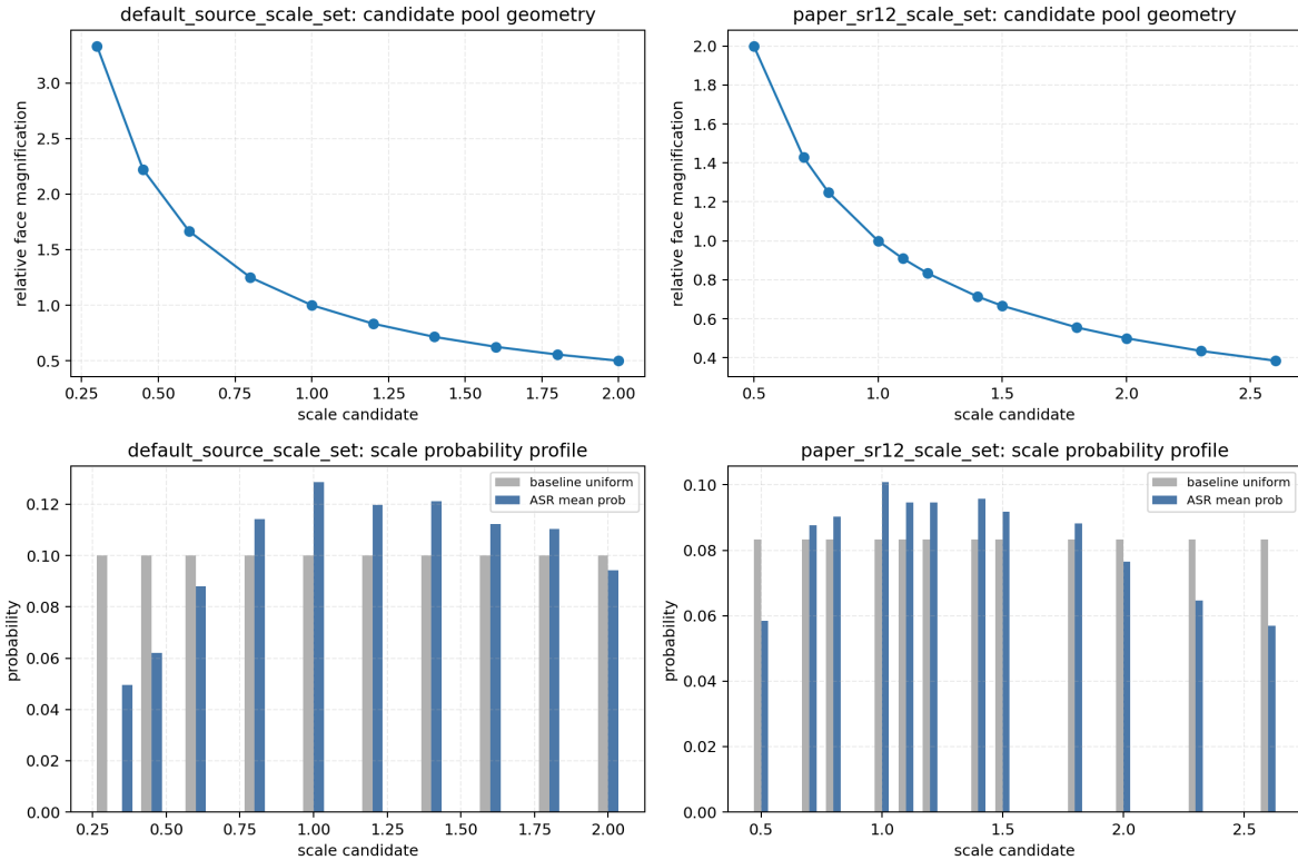
Hình III.8: So sánh hình học của hai tập tỉ lệ cắt và phân phối xác suất tương ứng.
