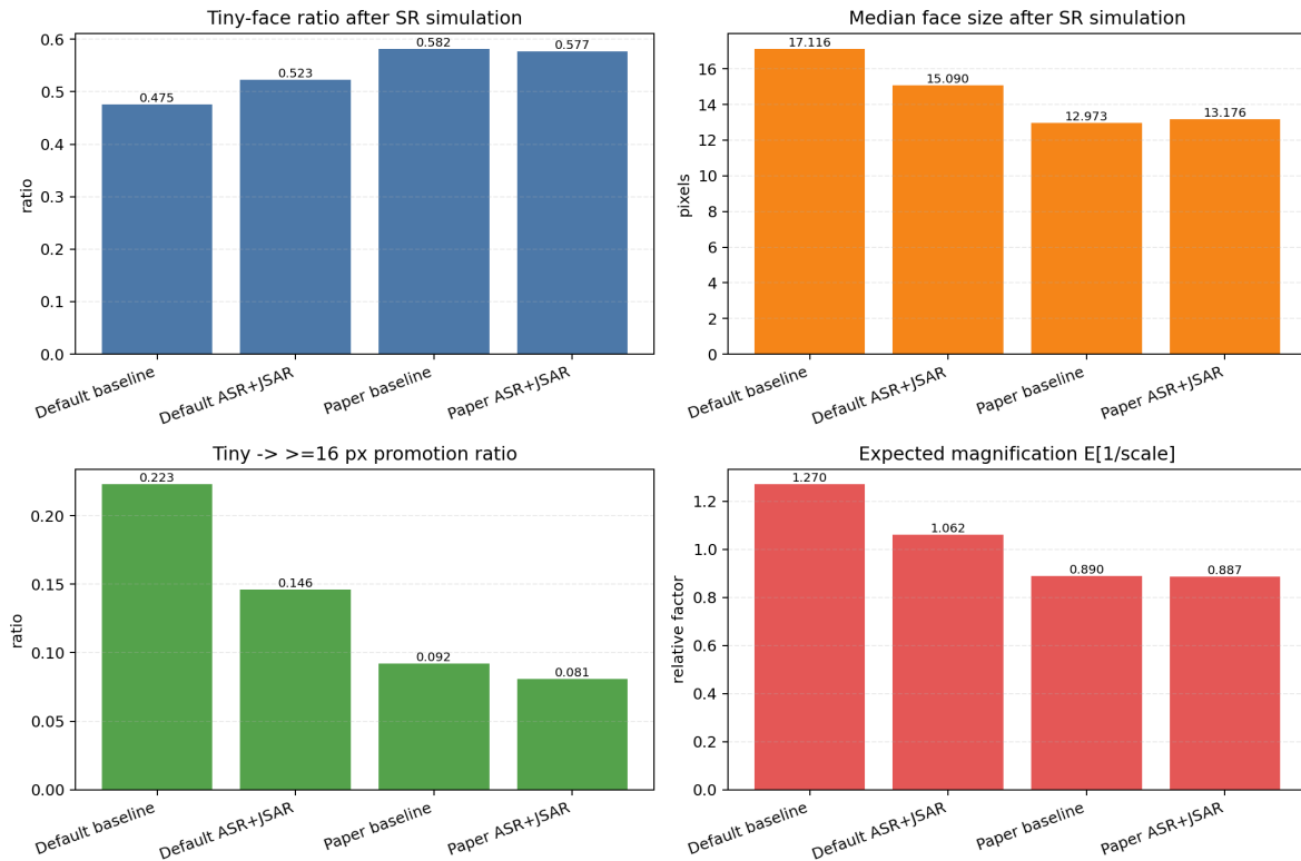
Hình III.9: So sánh phân phối kích thước khuôn mặt sau bước cắt và đổi cỡ ảnh giữa hai bộ tỉ lệ cắt.
