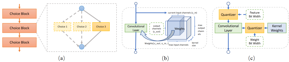
Hình VI.1: Minh họa luồng làm việc của SPOS (hình gốc từ bài báo SPOS [4]): (a) Tại mỗi stage có nhiều "khối lựa chọn", trong mỗi lượt truyền (forward pass), supernet sẽ chọn ngẫu nhiên một khối để kích hoạt; (b) Cơ chế cắt trọng số (weight slicing) được kích hoạt khi hai khối ở hai tầng liên tiếp có kích thước in/out khác nhau, khối lớn hơn sẽ tự động cắt bớt số kênh cho tương thích; (c) Kỹ thuật mixed precision [12] được tích hợp trong quá trình huấn luyện nhằm tối ưu bộ nhớ và thời gian.
